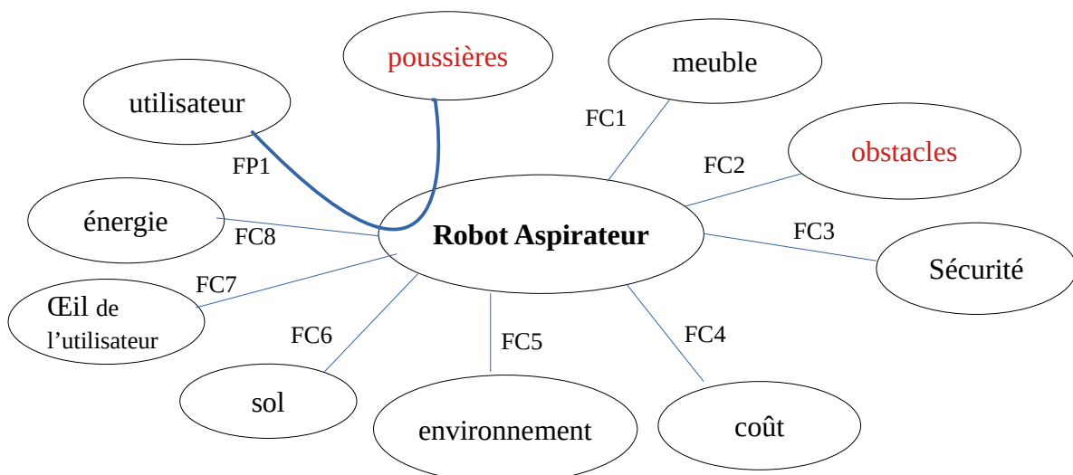
exemple du diagramme pieuvre pour un aspirateur robot
